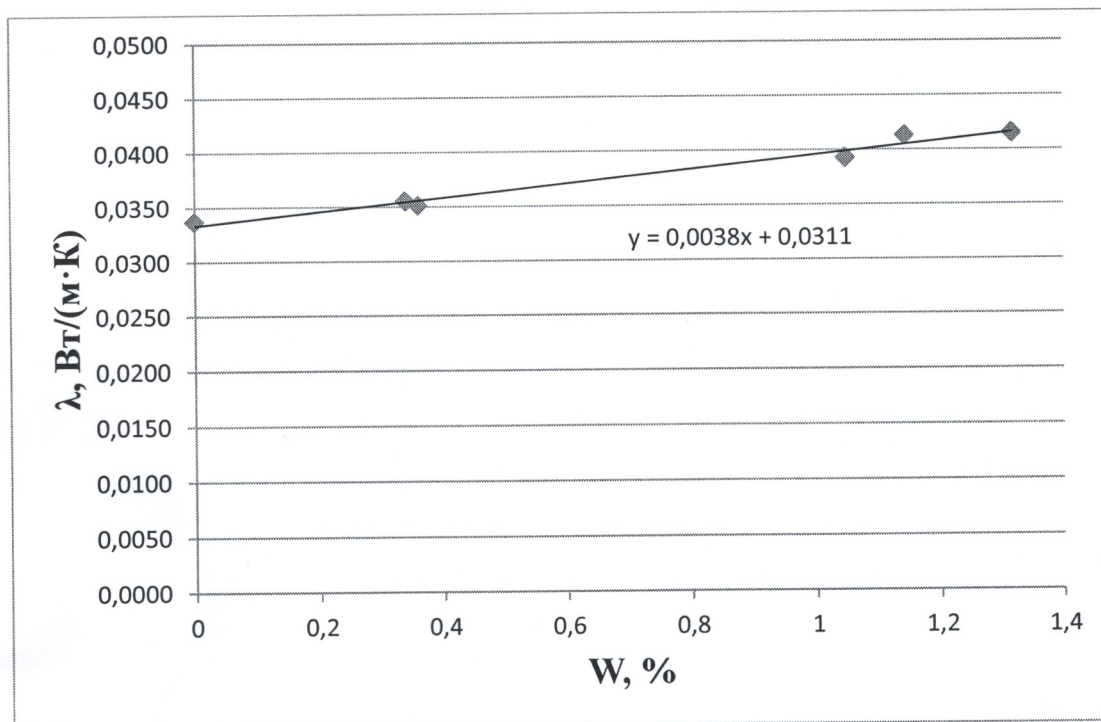
Рисунок 4 – Залежність теплопровідності при розрахунковій температурі матеріалу
